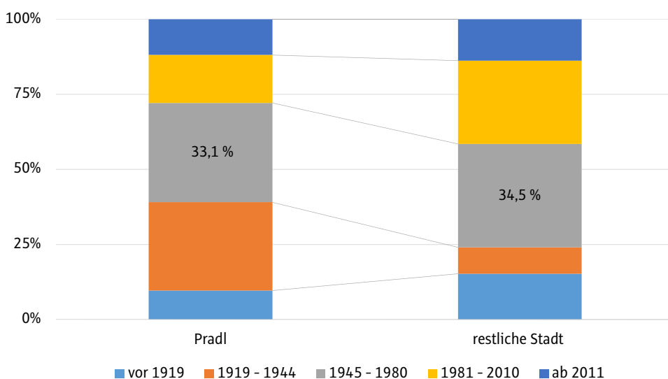
Gebäude nach Bauperiode
